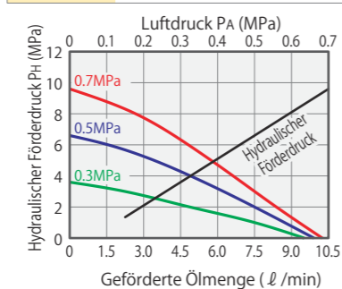
AC7001 Berechnungsformel PH = 60(PA - 0.06)
