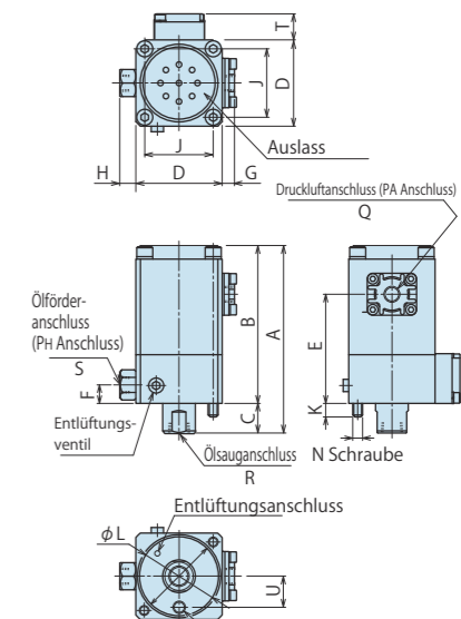
AC-V (Ventil, eingebaute Option)
