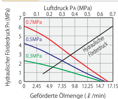
AC6001 Berechnungsformel PH = 37(PA - 0.06)
