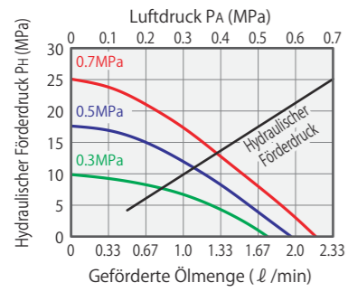
AB6000 Berechnungsformel PH = 38(PA - 0.04)
