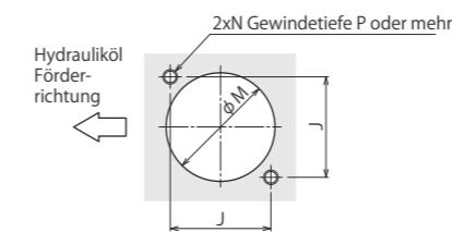
Fertigungsmaße für Montagebohrung (üblich)
