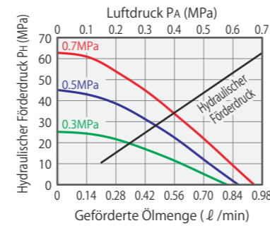
AB8000 Berechnungsformel PH = 95(PA - 0.04)
