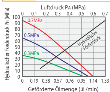
AC9001 Berechnungsformel PH = 147(PA - 0.06)
