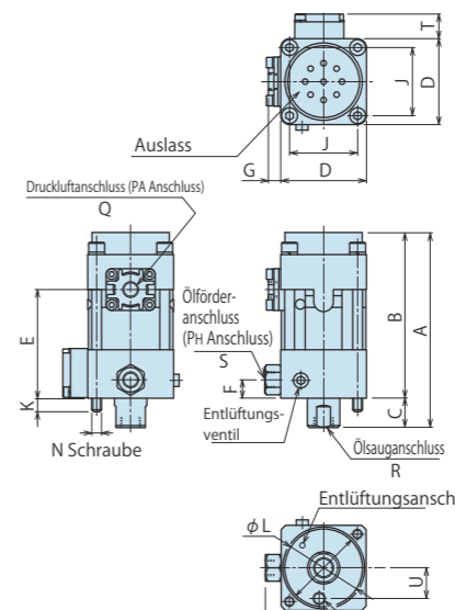
AB-V (Ventil, eingebaute Option)
