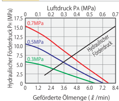
AC8001 Berechnungsformel PH = 94(PA - 0.06)
